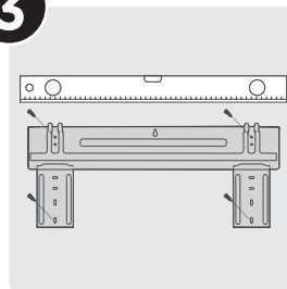
Определете позицията на отвора в стената
